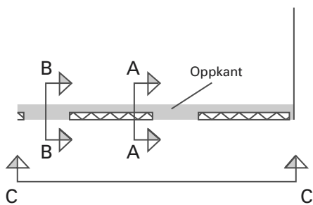
Typisk plan av kuldebrobryter i balkong
