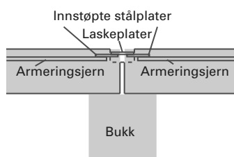
Typisk snitt igjennom stålplater
