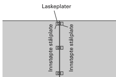
Typisk OK infesting av svalgang på underliggende bukk
