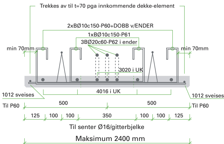
Tverrsnitt av slakkarmertbjelke
