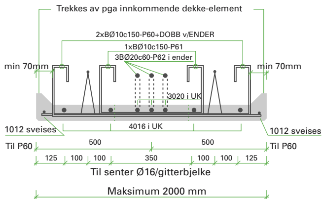
Tverrsnitt av slakkarmertbjelke med oppkanter
