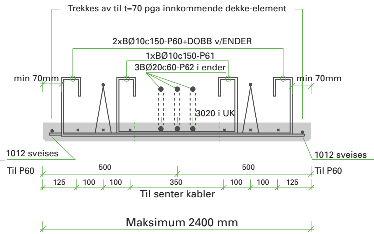
Tverrsnitt av forspent bjelke
