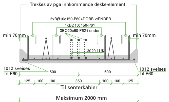
Tverrsnitt av forspentbjelke med oppkant
