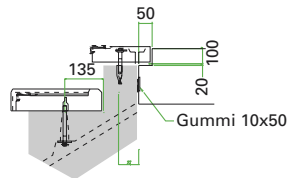
Opplegg oppe senterbjelketrapp
