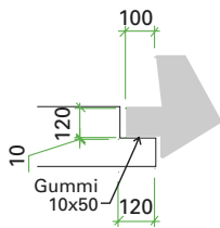
Opplegg nede platetrapp
