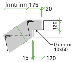
Opplegg oppe tettløpstrapp
