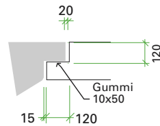
Opplegg oppe platetrapp
