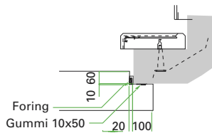
Opplegg nede senterbjelketrapp
