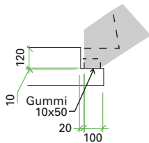
Opplegg nede tettløpstrapp
