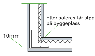
Innvendig hjørneløsning mellom 2 isolerte vegger
