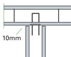
T-løsning med comax
