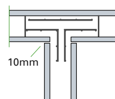
T-løsning ved veggskjøl/sliss
