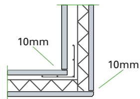
Utvendig hjørneløsning mellom 2 isolerte vegger
