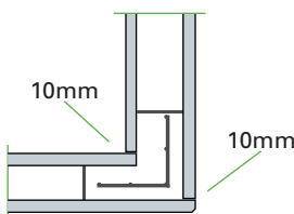
Utvendig hjørneløsning mellom 2 uisolerte vegger
