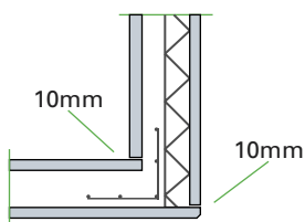
Hjørneløsning mellom isolert vegg og uisolert vegg
