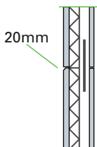
Horisontal fuge i isolert vegg
